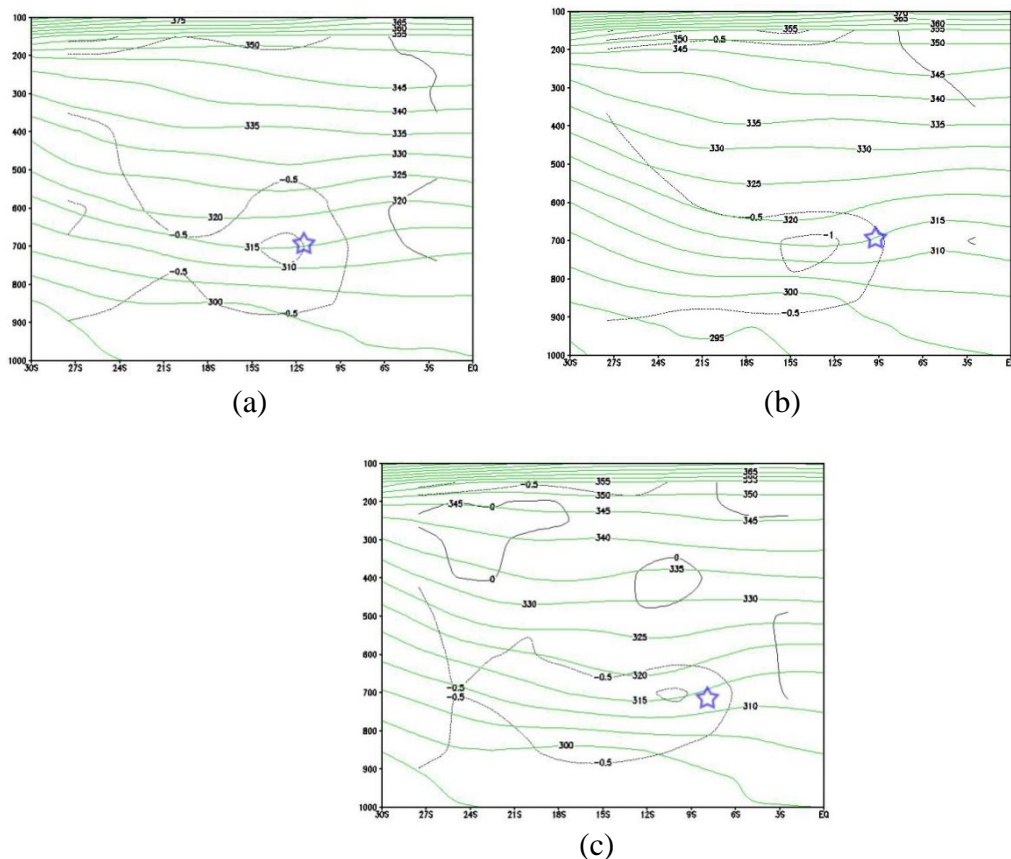
Figura 28 - Secção vertical em coordenada vertical de pressão, da temperatura potencial (K, em verde) e vorticidade potencial de Ertel (UVP, em preto) para: (a) 12/06/2008 às 18 UTC em 33°W; (b) 13/06/2008 às 12 UTC em 26°W; (c) 14/06/2008 às 12UTC em 29°W. A estrela em azul marca o centro do VCMN.
