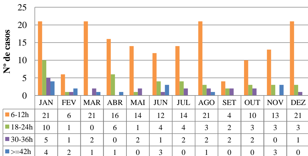
Gráfico 16 - Número de casos por mês e tempo de vida dos VCMN no ano de 2008.
